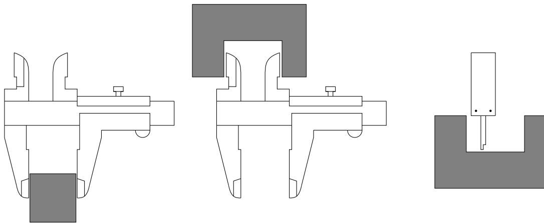
Kuva 1: Työntömitta.
