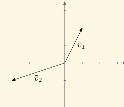
Kuva 5.4.1. Vektorit \mathbf{v}_1 ja \mathbf{v}_2 ovat lineaarisesti riippumattomia.
