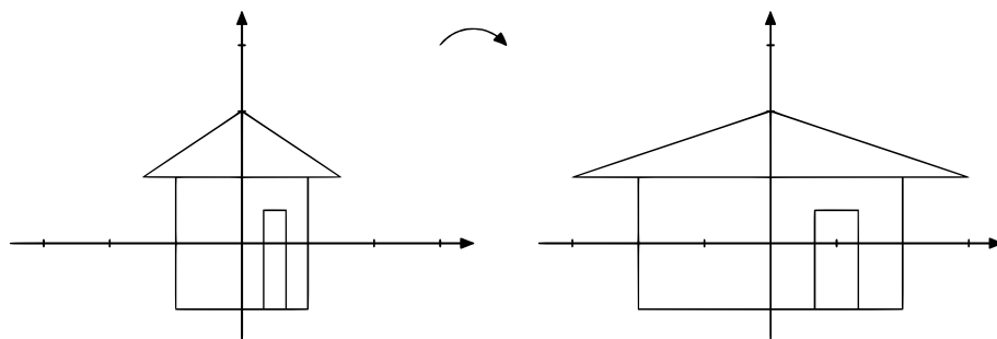
Kuva 3.3.1. Matriisi A venyttää vektoreita vaakasuunnassa.
