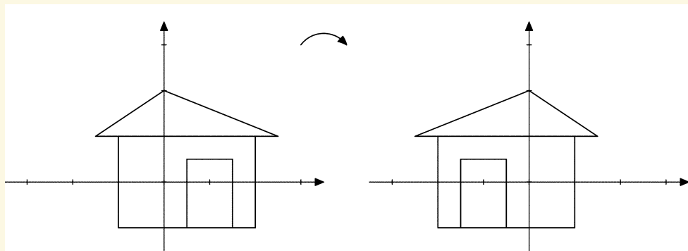
Kuva 6.4.1. Matriisi B peilaa vektorit vaak akselin suhteen.
