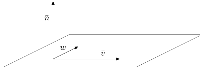
Kuva 2.2.4. Tason normaali \mathbf{n} .
