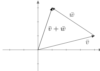
Kuva 1.2.1. Vektorit \mathbf{v} ja \mathbf{w} sekä niiden summa \mathbf{v} + \mathbf{w} .
