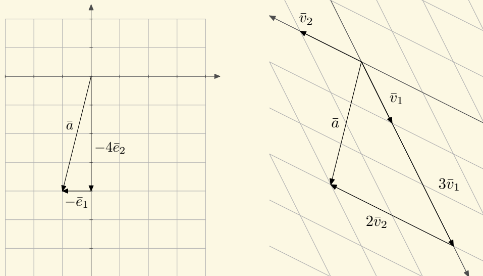
Kuva 5.5.2. Vektori \mathbf{a} luonnollisen kannan \mathcal{E}_2 määräämässä koordinaatistossa ja kannan \mathcal{B} määräämässä koordinaatistossa. Kun käytetään jotakin muuta kuin luonnollista kantaa, vääntyy koordinaatisto vinoon.
