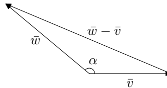
Kuva 1.3.2. Vektoreiden \mathbf{v} ja \mathbf{w} välinen kulma kosinilauseen näkökulmasta.
