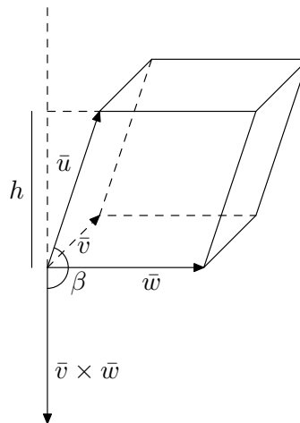
Kuva 1.5.5. Vektoreiden \mathbf{v} , \mathbf{w} ja \mathbf{u} määrämän suuntaissärmiön tilavuus.
