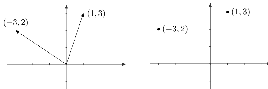
Kuva 1.1.1. Vektoreita (1, 3) ja (-3, 2) voi havainnollistaa origosta lähtevänä nuolena tai koordinaatiston pisteinä.
