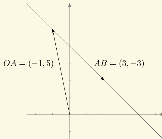
Kuva 2.1.5. Suora S = \{(-1, 5) + t(3, -3) \mid t \in \mathbb{R}\} .
