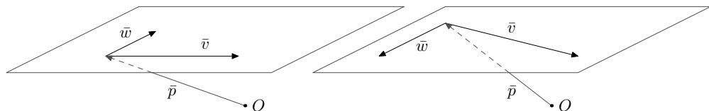
Kuva 2.2.3. Taso voidaan kirjoittaa eri tavoin joukkona \{\mathbf{p} + s\mathbf{w} + t\mathbf{v} \mid s, t \in \mathbb{R}\} .
