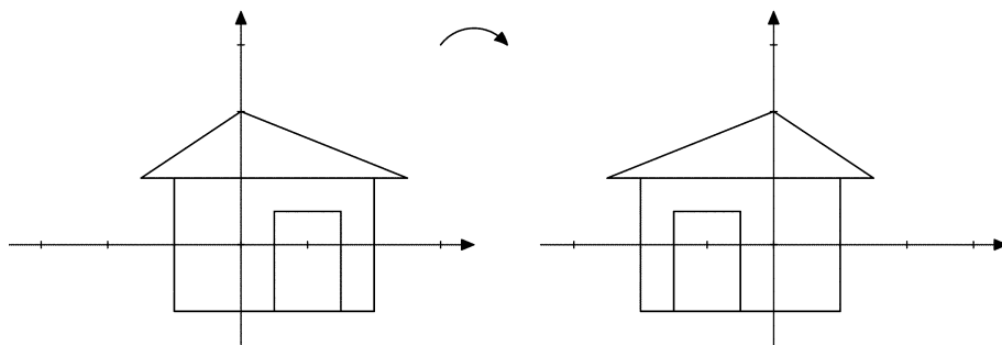
Kuva 3.3.2. Matriisi B peilaa vektorit pystyakselin suhteen.
