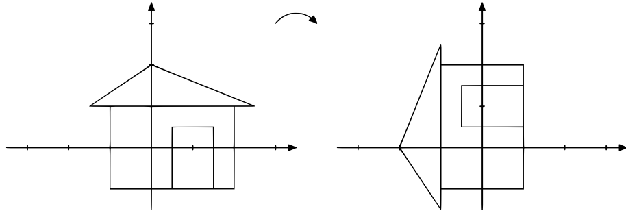
Kuva 3.3.3. Matriisi C kiertää vektoreita kulman \pi/2 verran positiiviseen kiertosuuntaan.
