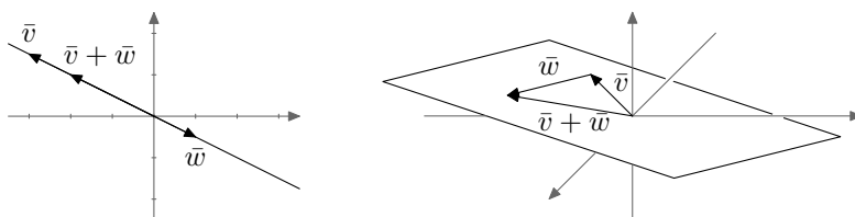
Kuva 16.50: Esimerkiksi origon kautta kulkevat suorat ja tasot ovat avaruuden \mathbb{R}^3 aliavaruuksia. Ne ovat suljettuja yhteenlaskun (kuvassa) ja skalaarikertolaskun suhteen.
