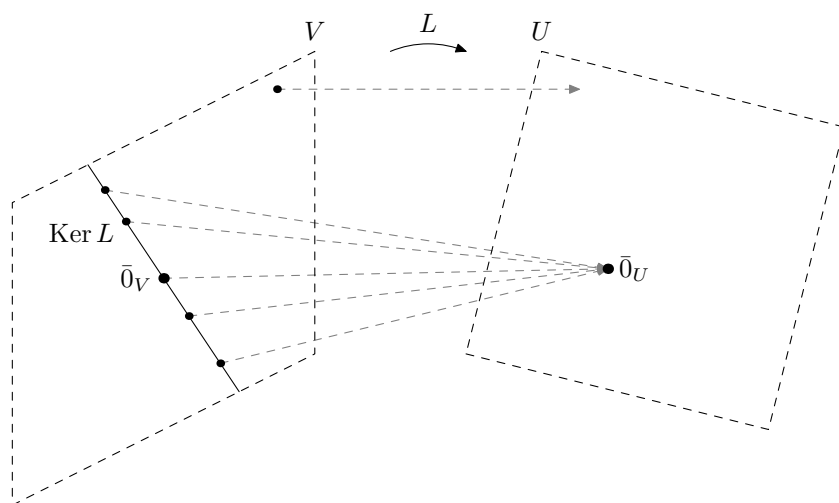
Kuva 20.64: Lineaarikuvauksen L ydin koostuu kaikista niistä vektoreista, jotka kuvautuvat nollavektorille.
