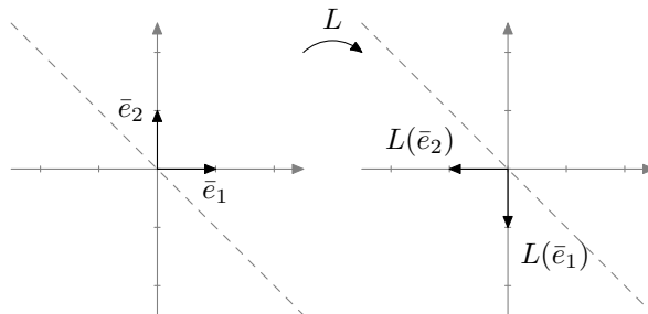
Kuva 22.69: Kantavektorien \bar{e}_1 ja \bar{e}_2 kuvautuminen lineaarikuvauksessa L .
