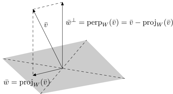
Kuva 24.88: Vektori \bar{v} voidaan kirjoittaa summana vektoreista, jotka ovat aliavaruuksien W ja W^\perp alkioita.
