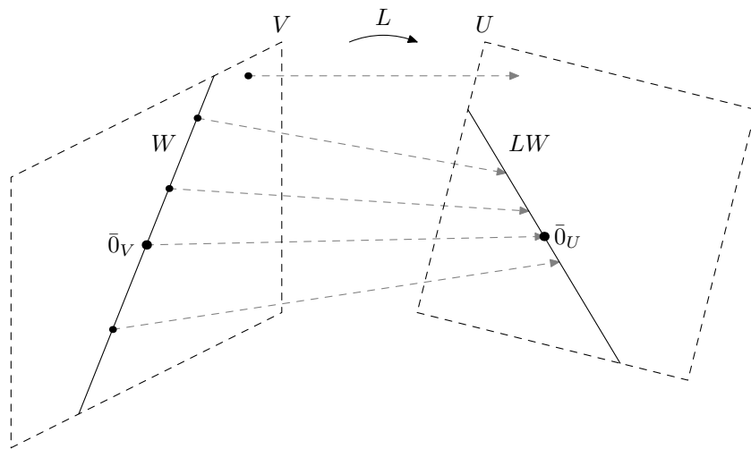
Kuva 19.61: Aliavaruuden W kuva lineaarikuvauksessa L on maaliavaruuden osajoukko.
