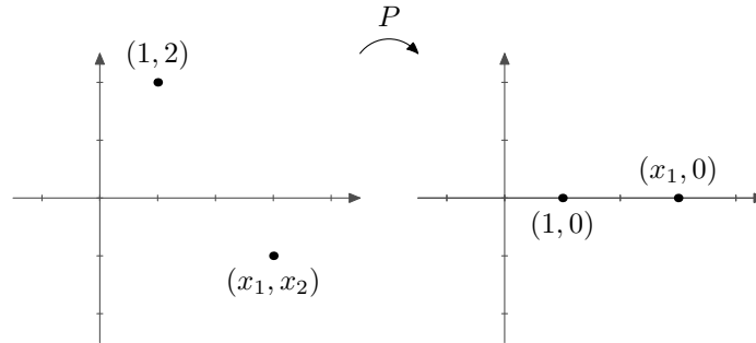
Kuva 19.59: Kuvaus P projisoi vektorit vaaka-akselille.
