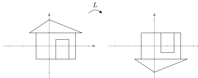
Kuva 19.62: Lineaarikuvaus L peilaa vektorit vaaka-akselin suhteen.
