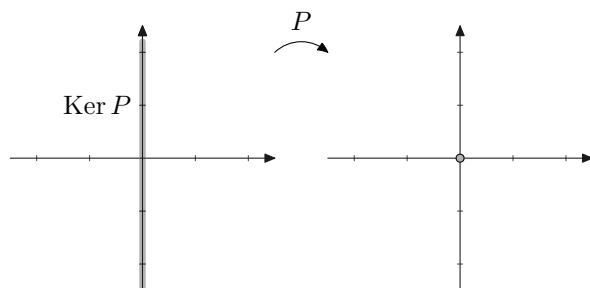
Kuva 20.65: Lineaarikuvarauksen P ytimen vektorit kuvautuvat nollavektoriksi.
