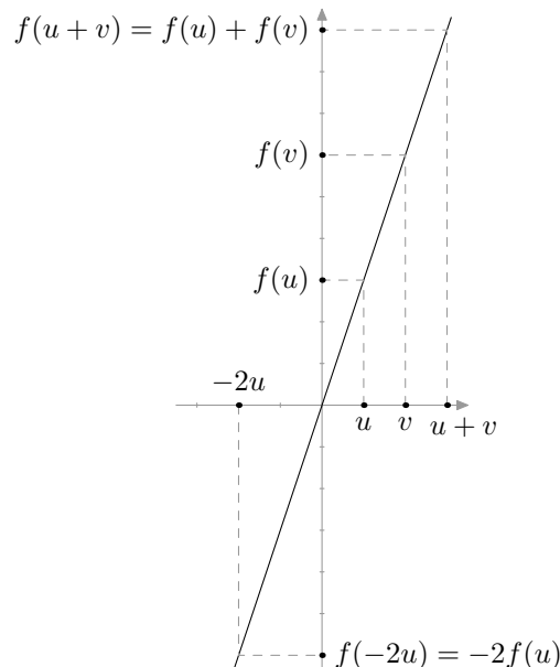
Kuva 19.54: Kuvaus f täyttää lineaarikuvauksen määritelmän ehdot.
