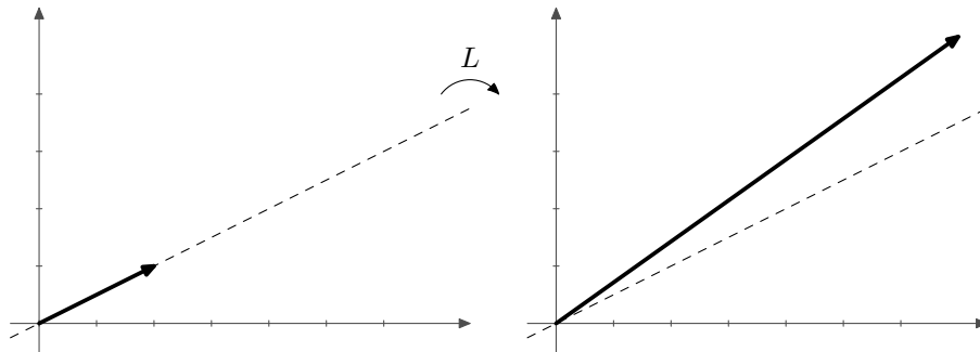
Kuva 23.74: Vektori (2, 1) ei ole lineaarikuvauksen L ominaisvektori.
