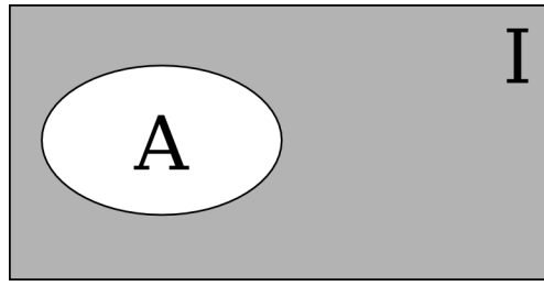
KUVA 6. Joukon A komplementti, I \setminus A
